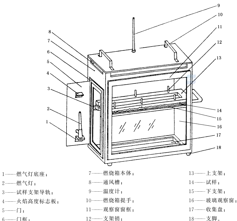
图 1 燃烧箱
