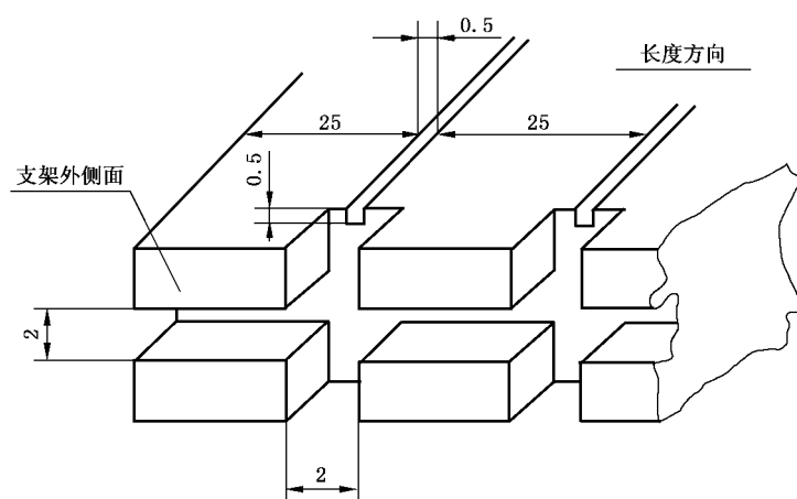
图 5 下支架截面图
