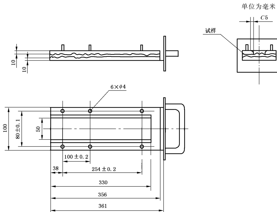
图 4 试样支架
